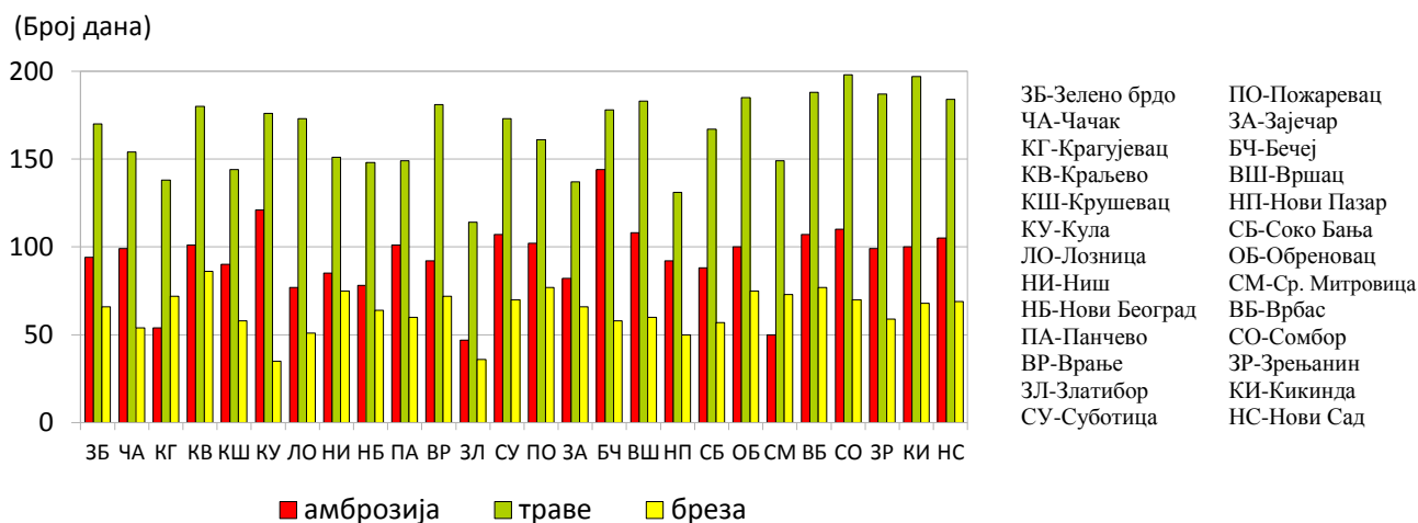
Слика 31. Број дана са присутном полинацијом за све станице у Републици Србији у 2017. години
