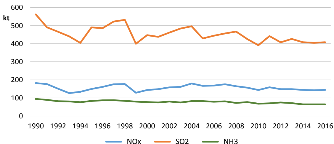
Слика 4. Емитоване количине закисељавајућих гасова у Републици Србији у периоду 1990 – 2016. година (kt/год)
