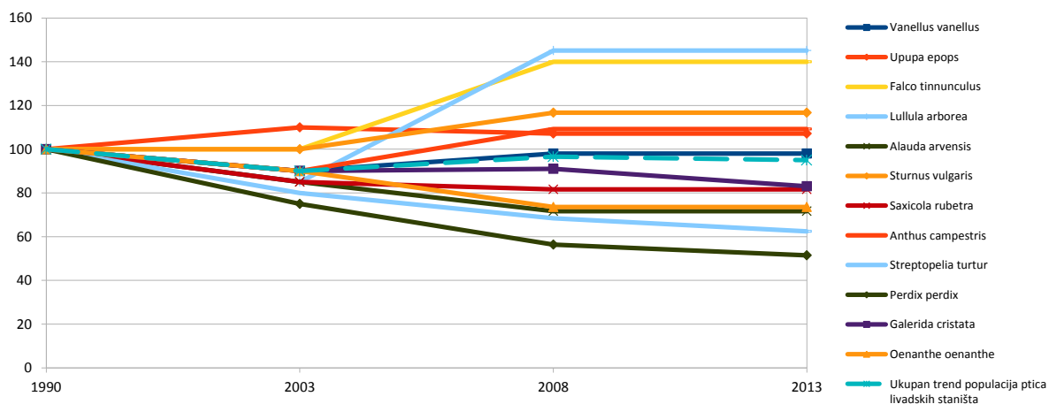
Слика 73. Тренд популација ливадских врста птица (12 врста)
