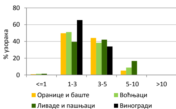
Слика 80. Садржај хумуса (%)
