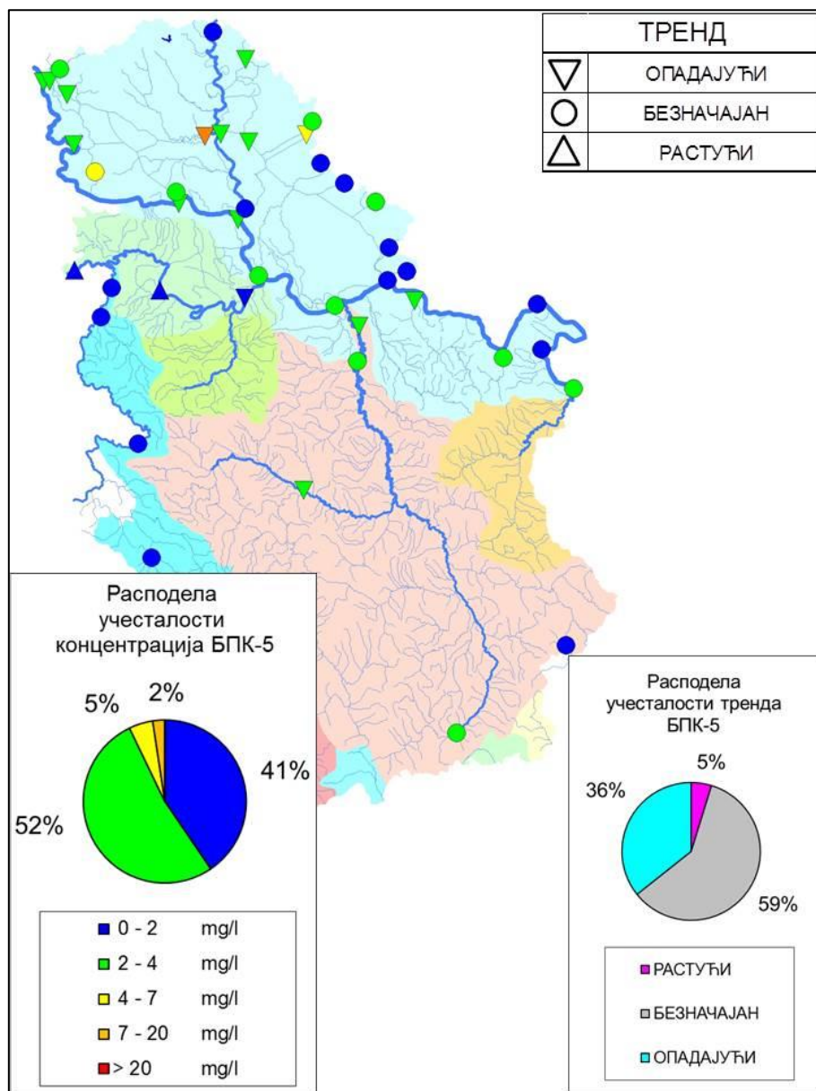
Слика 37. Тренд и средња вредност концентрација БПК-5 у водотоцима Републике Србије (2007-2016.)
