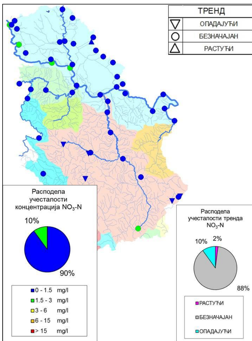
Слика 43. Тренд и средња вредност концентрација нитрата у водотоцима Републике Србије (2007-2016.)
