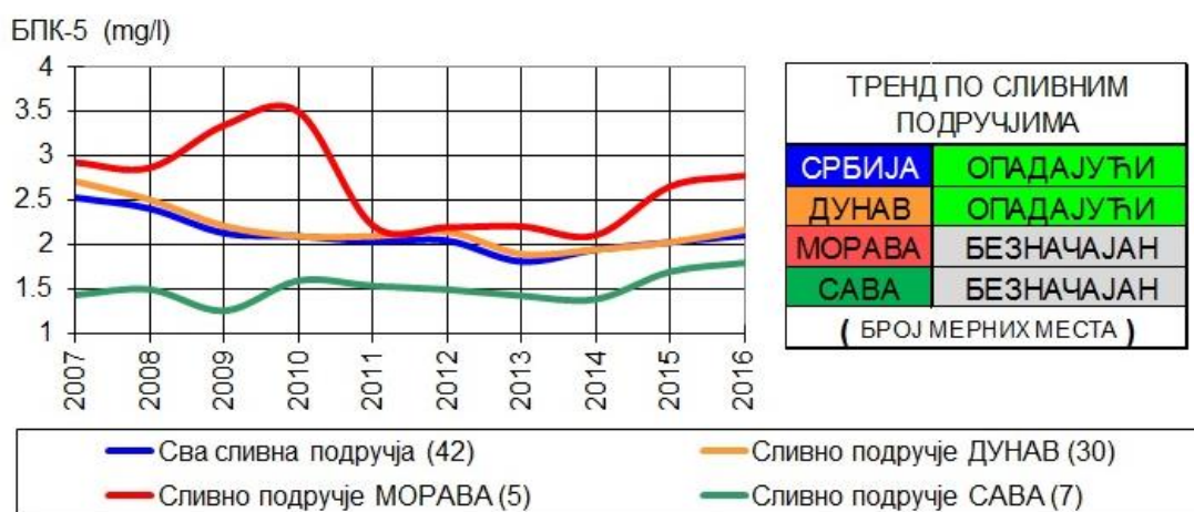
Слика 36. Трендови медијана БПК-5 у сливним подручјима Републике Србије (2007-2016.)
