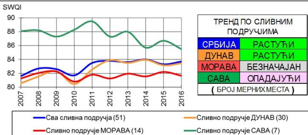
Слика 48. Трендови медијана SWQI у сливним подручјима Републике Србије (2007-2016.)
