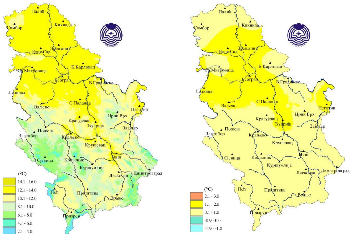
Слика 34. Распореда годишњих вредности температуре (лево) на подручју Републике Србије у 2017. години и одступања средње годишње температуре у (°C) од нормале 1981-2010. (десно)
