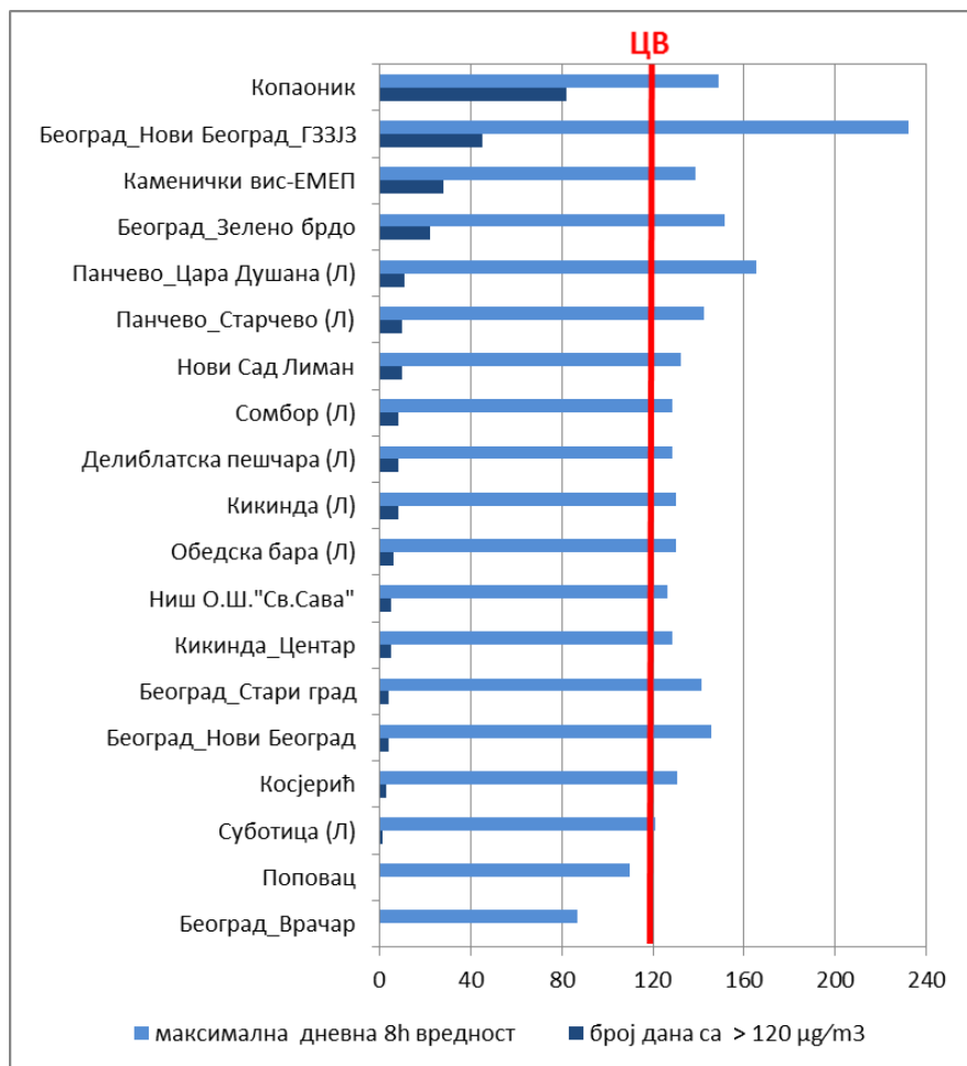
Слика 28. Упоредни приказ максималних дневних осмосатних концентрација O_3 ( \mu\text{g}/\text{m}^3 ) и броја дана са прекорачењем ЦВ у 2019. години
