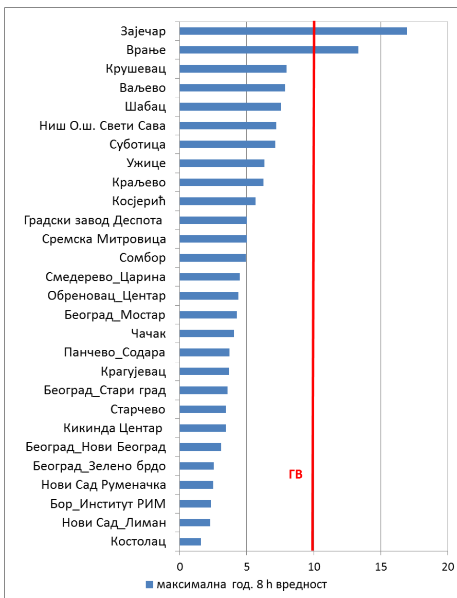
Слика 30. Приказ максималних осмосатних концентрација СО (mg/m 3 ) у 2019. години
