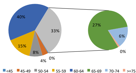
Слика 99. Процентуална расподела укупног индикатора буке L_{den} за анализиране градове Републике Србије
