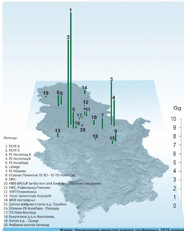
Слика 2. Емисије оксида азота
