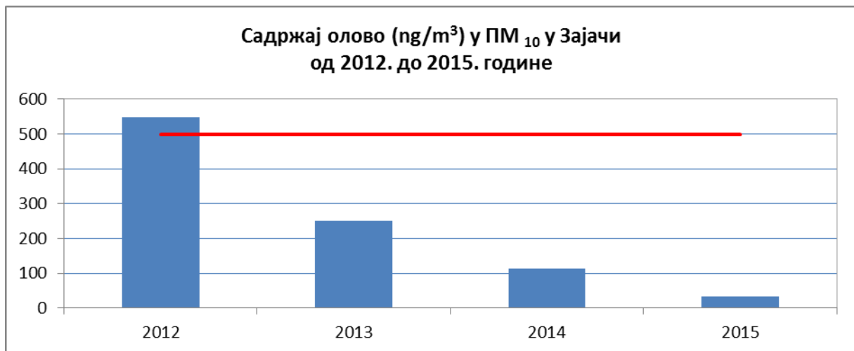
Слика 1. Средње годишње концентрације олова у суспендованим честицама \text{PM}_{10} у Зајачи у периоду 2012.- 2015. година.
