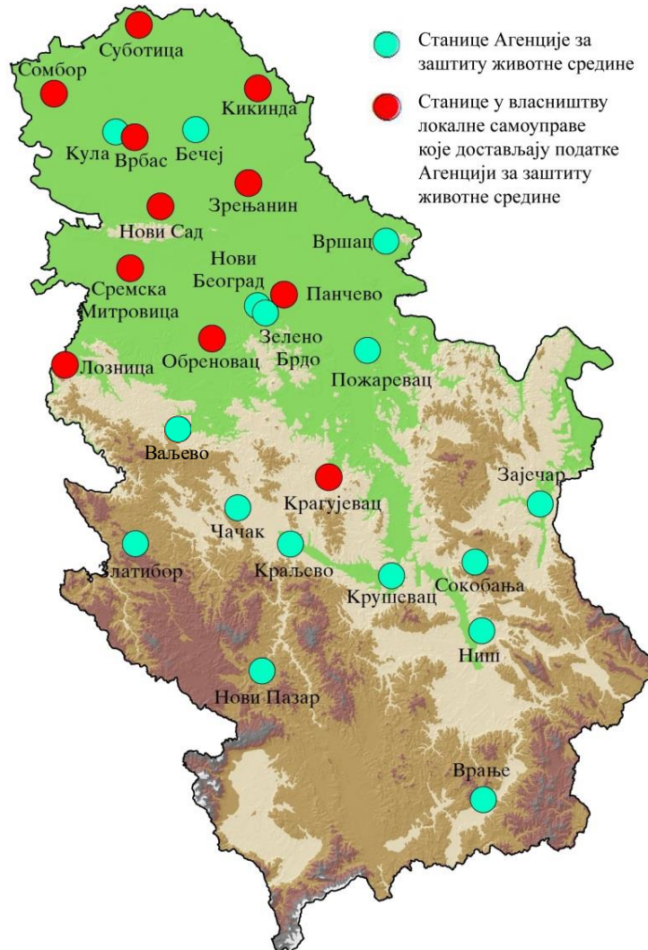
Слика 28. Мрежа станица за праћење алергеног полена
