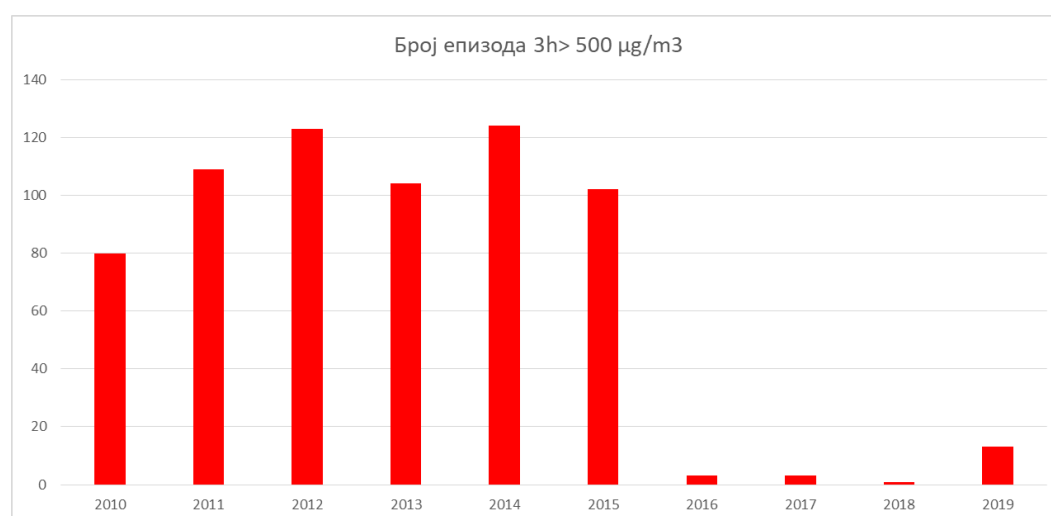
Слика 17. Број епизода са прекорачењем вредности концентрација \text{SO}_2 већих од 500\mu\text{g}/\text{m}^3 три или више сати заредом у Бору (Градски парк) у периоду од 2010. до 2019. године
