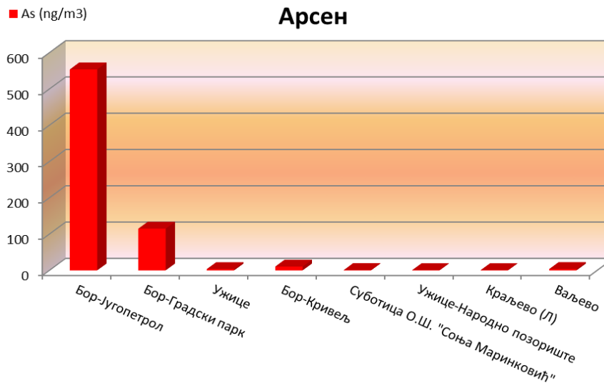
Слика 1. Средња годишња вредност арсена у 2019. години
