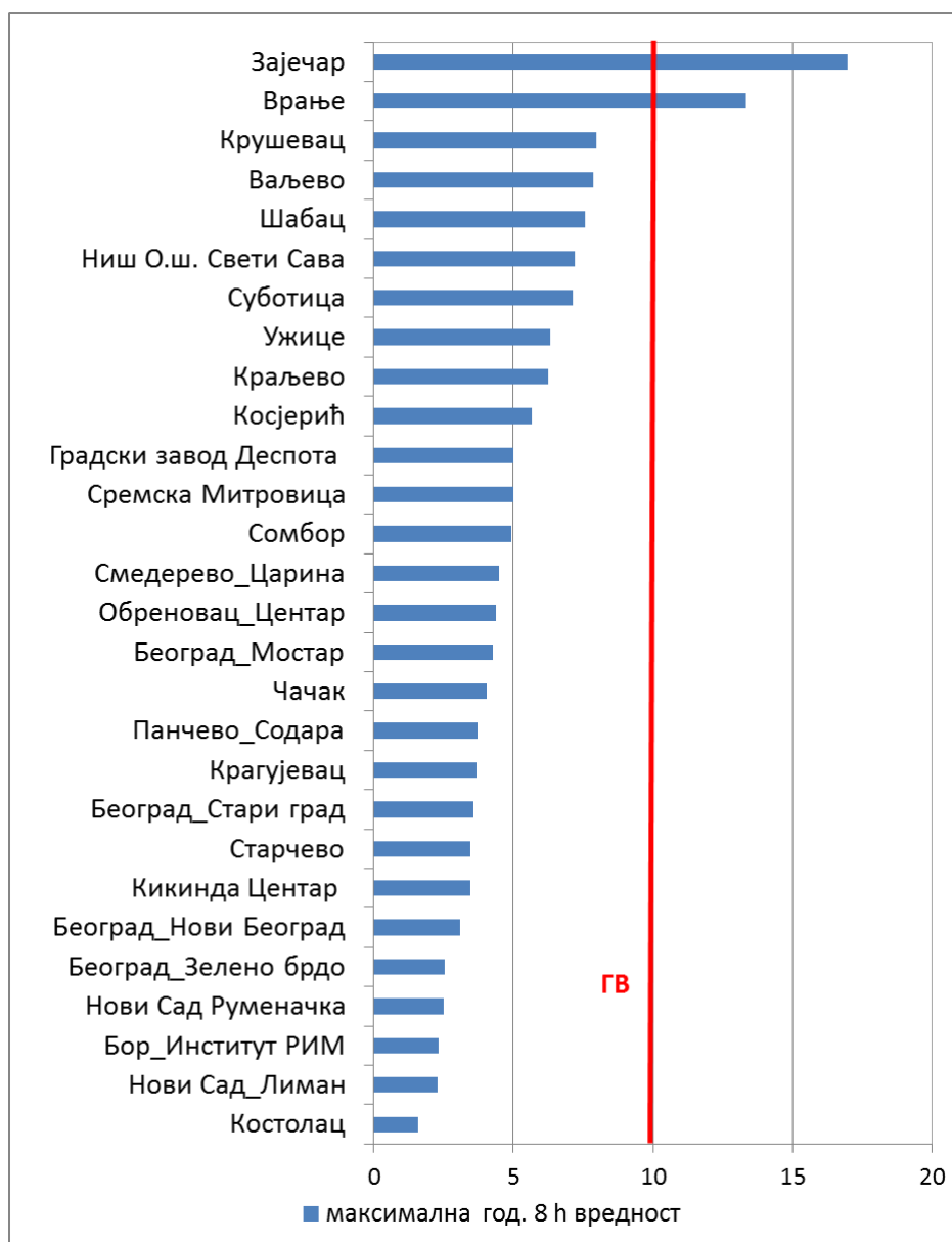
Слика 30. Приказ максималних осмосатних концентрација СО ( \text{mg}/\text{m}^3 ) у 2019. години
