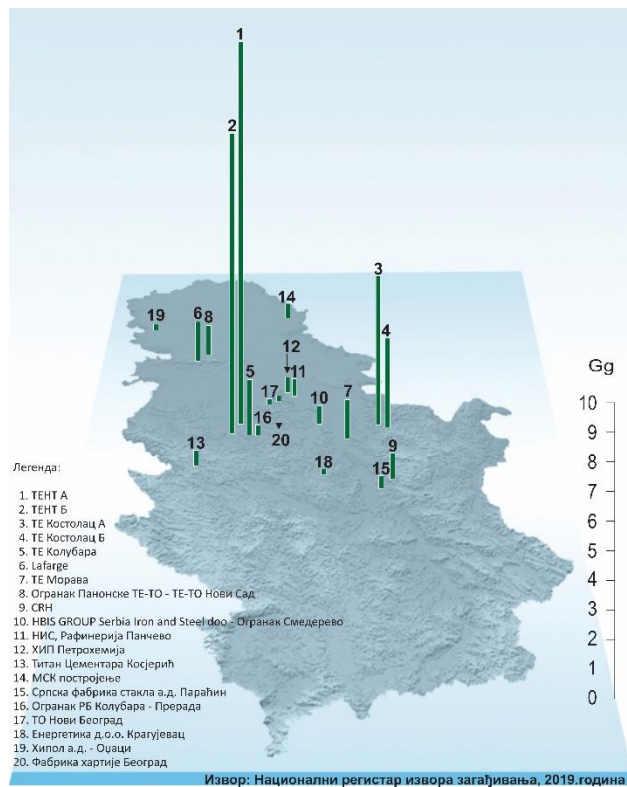
Слика 2. Емисије оксида азота
