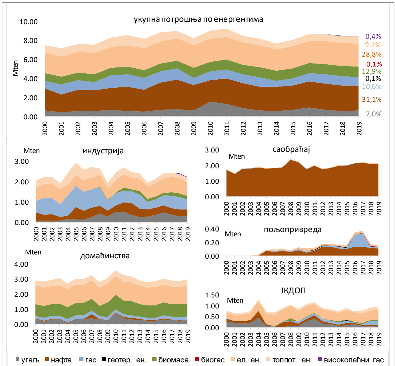
Слика 161. Потрошња финалне енергије по енергентима укупно и у секторима у Републици Србији
