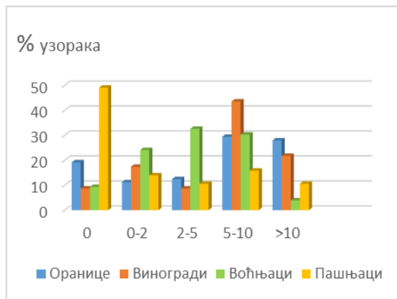
Слика 90. Садржај CaCO 3 (%)
