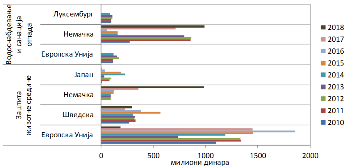
Слика 183. Највећи донатори за секторе „Заштита животне средине” и „Водоснабдевање и санација отпада”
