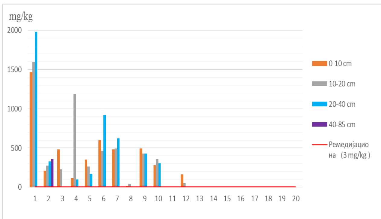
Слика 98. Прекорачење садржаја антимиона у проучаваним земљиштима
