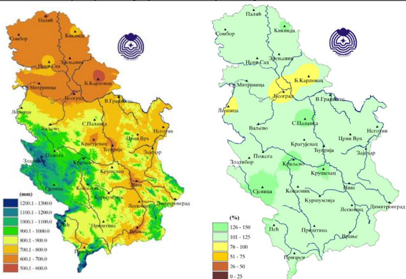
Слика 38. Распореда количина падавина (десно) на подручју Републике Србије у 2018. години (лево) и одступања годишње количине падавина у процентима од нормале 1981-2010.
