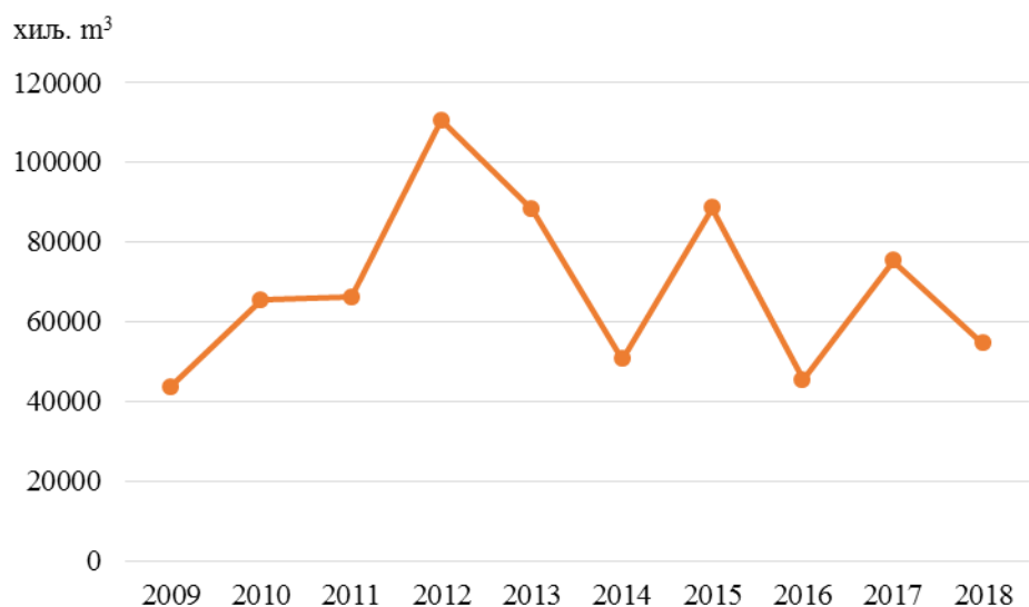
Слика 164. Захваћене воде за наводњавање пољопривредних површина (хиљада m³)
