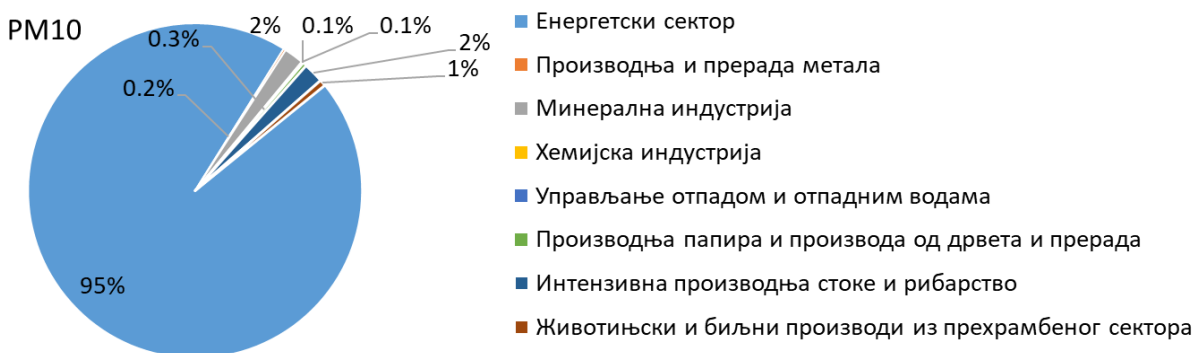
Слика 2.3. Емисије прашкастих материја
