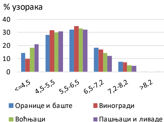
Слика 5.2. Супституционална киселост (pH у nKCl-у)
