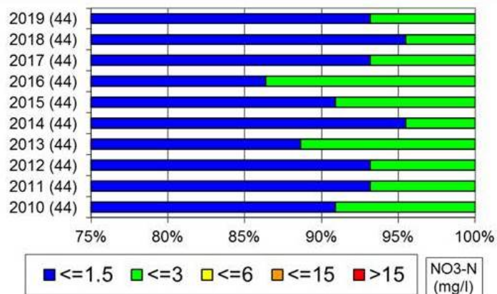
Слика 3.9. Расподела учесталости нитрата у водотоцима Републике Србије (2010-2019. године)
