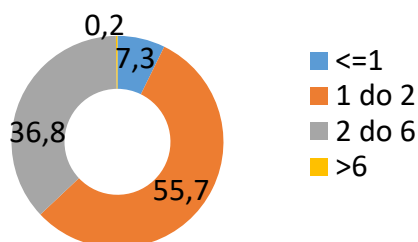
Слика 5.7. Садржај органског угљеника (ОС)
