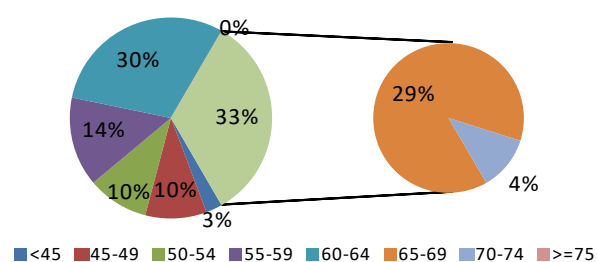
Слика 7.2. Процентуална расподела укупног индикатора буке L_{den} за анализирани градове Републике Србије
