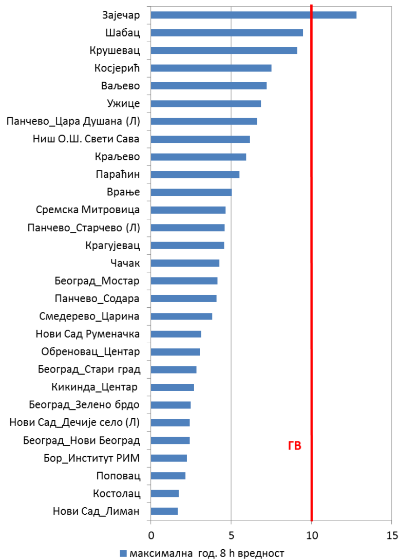
Слика 2.29. Приказ максималних осмосатних концентрација CO (mg/m 3 ) у 2020. години
