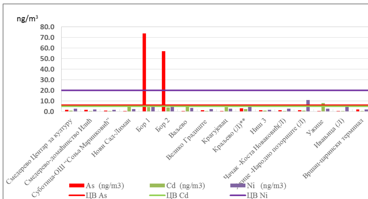
Слика 9. Средње годишње вредности арсена, кадмијума и никла добијене индикативним мерењима у 2018. години (ng/m 3 ) и прописане циљне вредности
