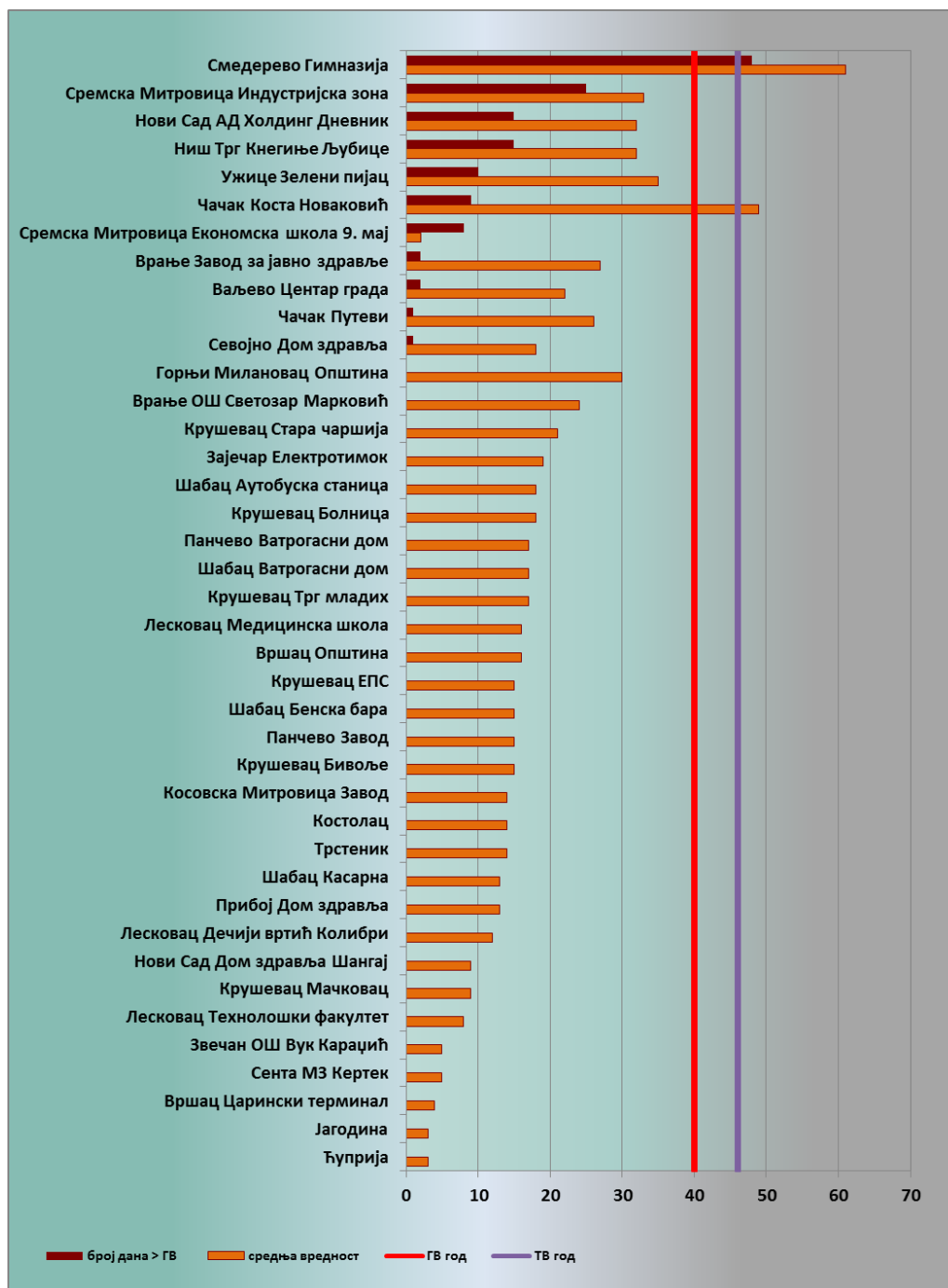
Слика 25. Средња годишња концентрација NO 2 (µg/m 3 ) и број дана са прекорачењем ГВ у 2018. години
