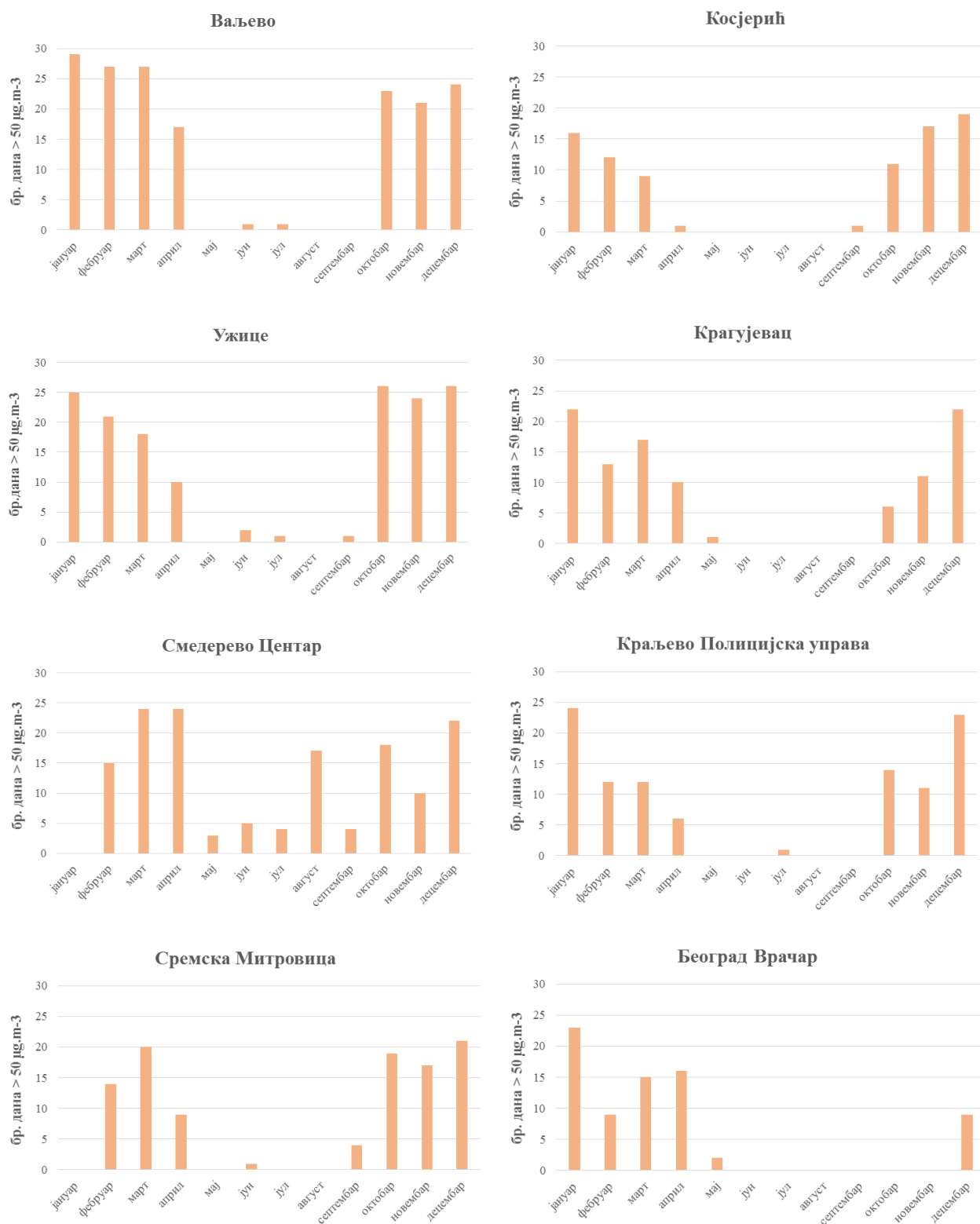
Слика 8. Приказ броја дана са прекорачењем дневне ГВ PM_{10} ( \mu g/m^3 ) по месецима у 2018. години
