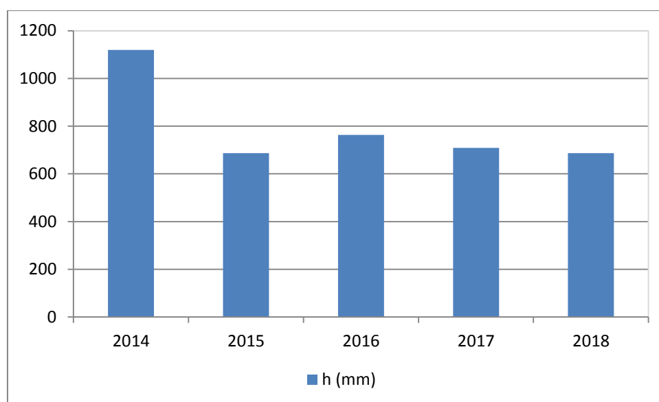
Слика 15. Тренд годишње суме падавина на станици Каменички Вис
