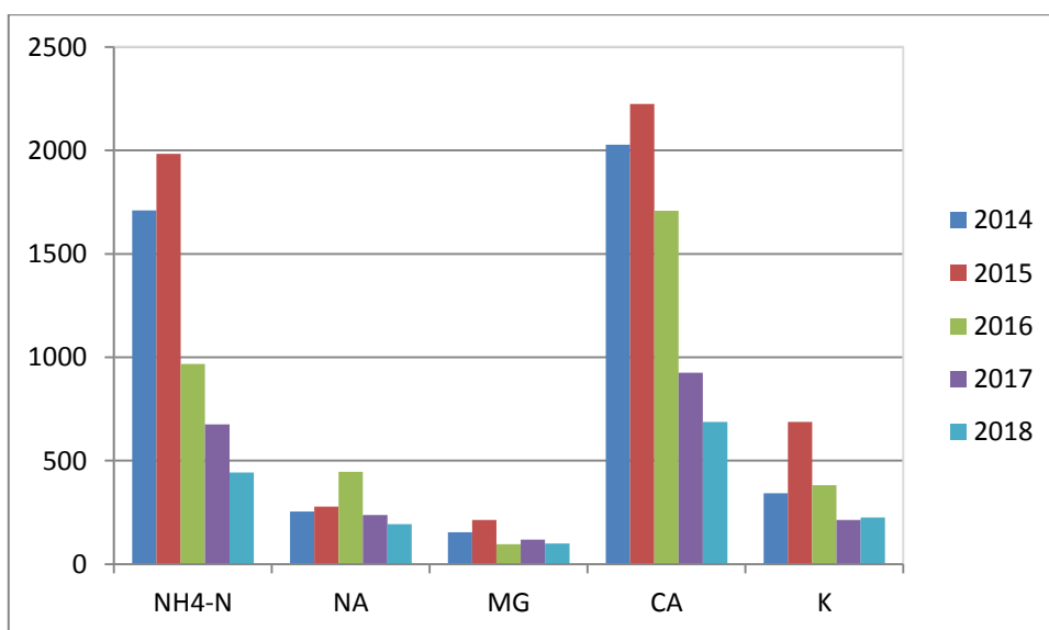
Слика 17. Тренд депозиција азота из амонијум јона, натријума, магнезијума, калцијума и калијума
