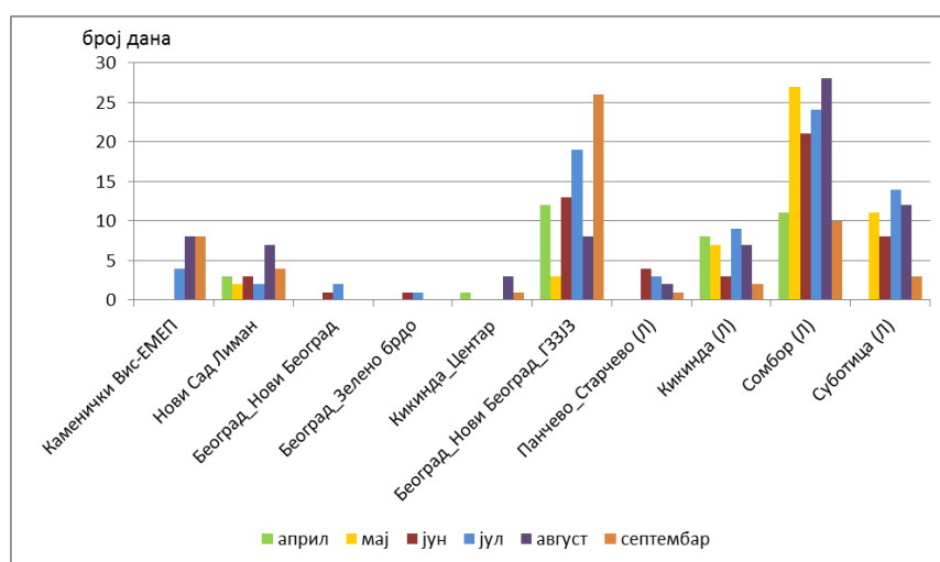
Слика 14. Приказ броја дана са прекорачењем ЦВ \text{O}_3 у сезони април-септембар 2018. године
