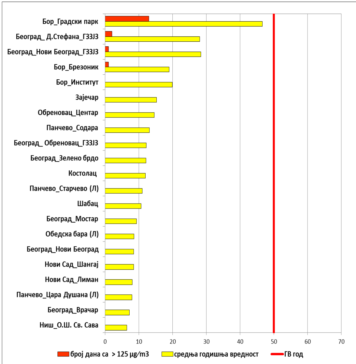
Слика 5. Упоредни приказ средње годишње концентрације \text{SO}_2 ( \mu\text{g}/\text{m}^3 ) и броја дана са прекорачењем ГВ у 2018. години
