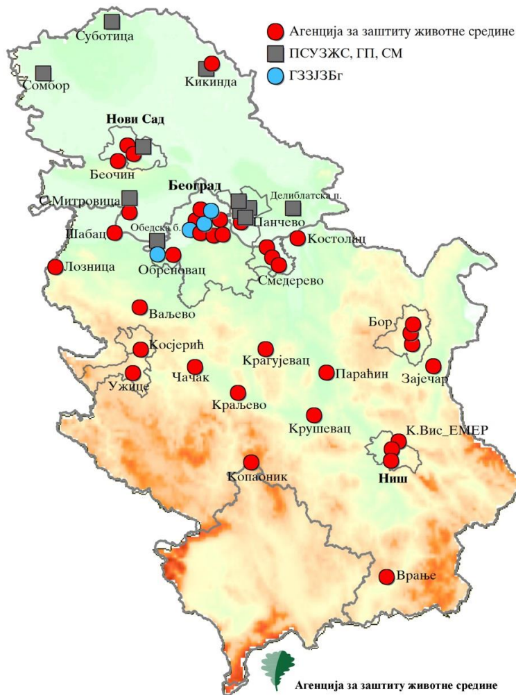
Слика 1. Мреже станица за квалитет ваздуха Агенције за заштиту животне средине, Градског завода за јавно здравље Београда, ПСУЗЖС Војводине, градова Панчева, Сремске Митровице и Краљева
